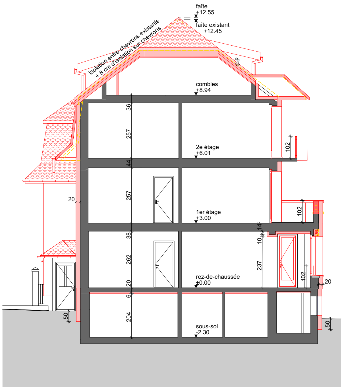
COUPE B-B
