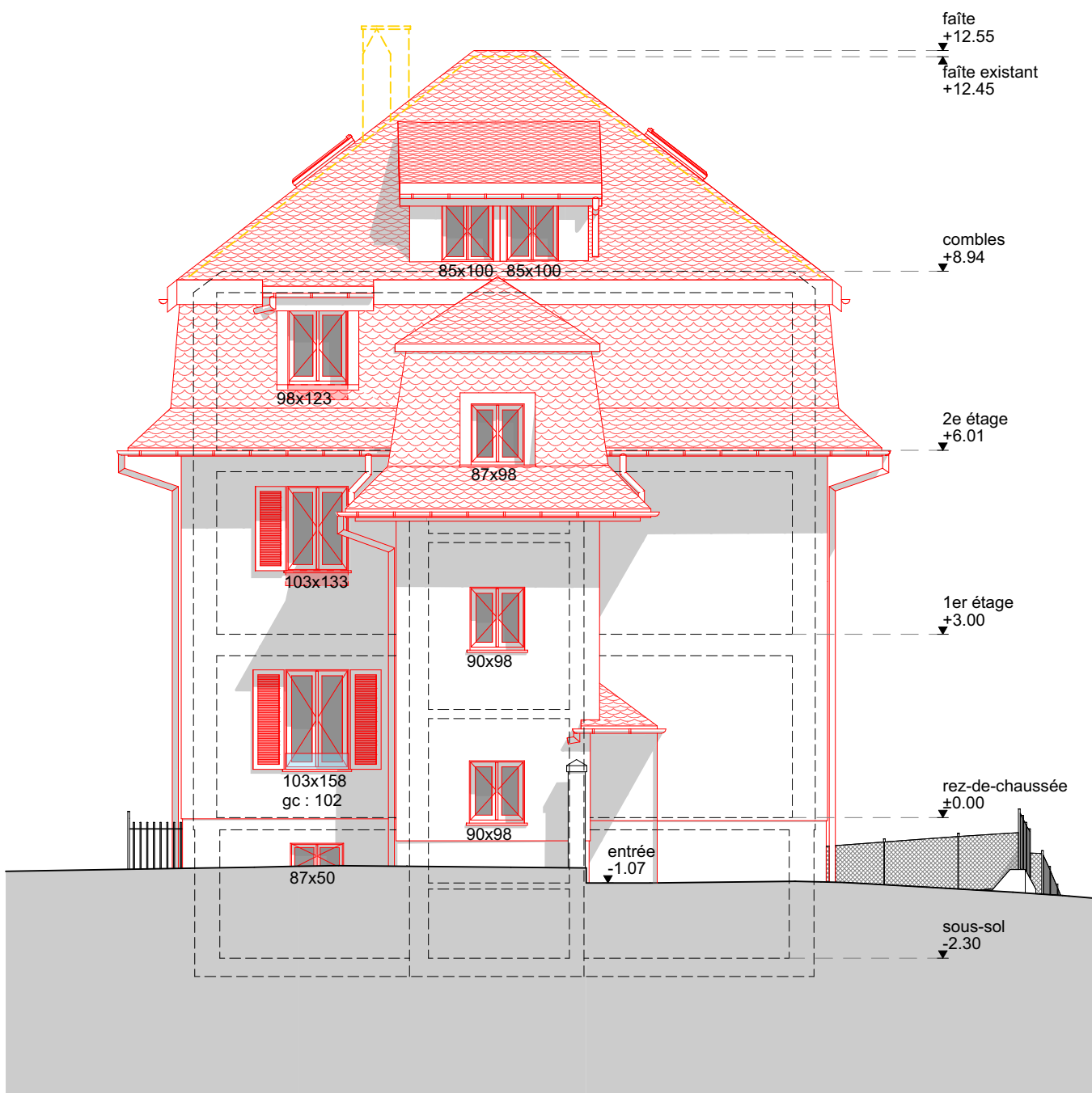
FACADE EST
