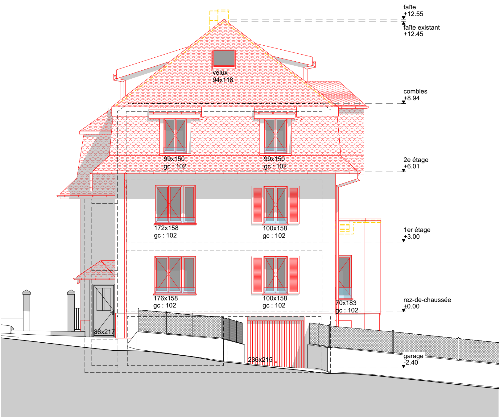
FACADE NORD
