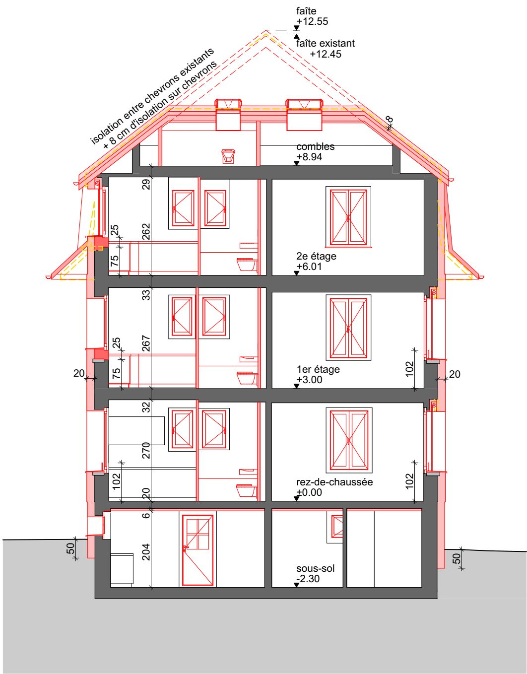
COUPE A-A
