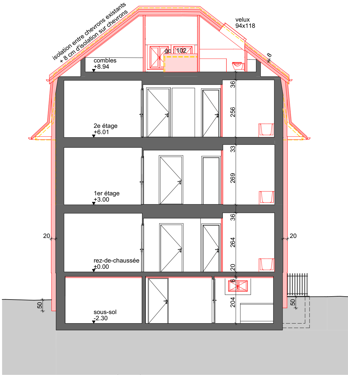
COUPE C-C
