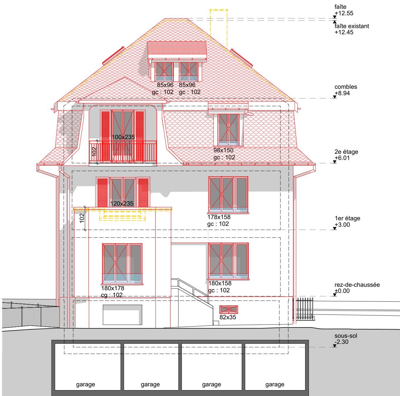
FACADE OUEST
