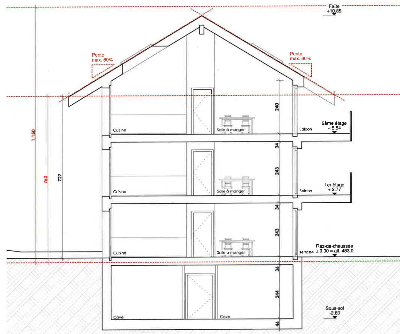
Coupe A-A
