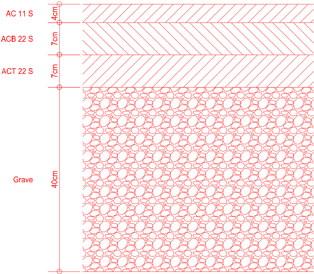
Coupe type 1:4 Structure de couche d'enrobé nouveau
