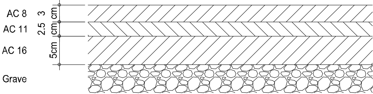
Coupe type 1:4 Structure de couche d'enrobé existant
